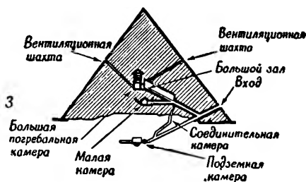
Схематические разрезы пирамид. 1. Пирамида Снофру. 2. Пирамида Хефрена. 3. Пирамида Хеопса
