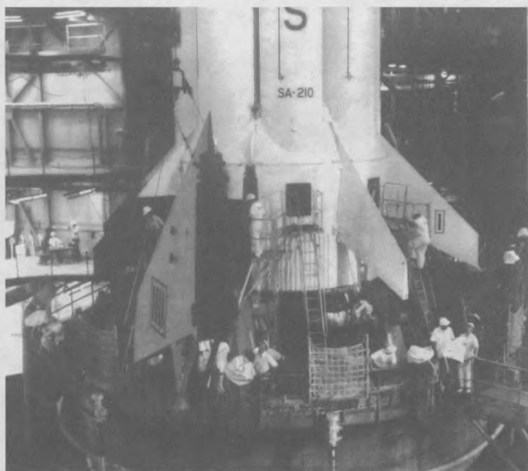
Сборка ракеты-носителя в космическом центре им. Джонсона. Хьюстон, США. 1975 г.
