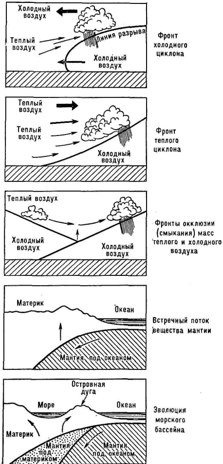
Рис. 5. Сравнение движения потоков циклона и вещества мантии.
