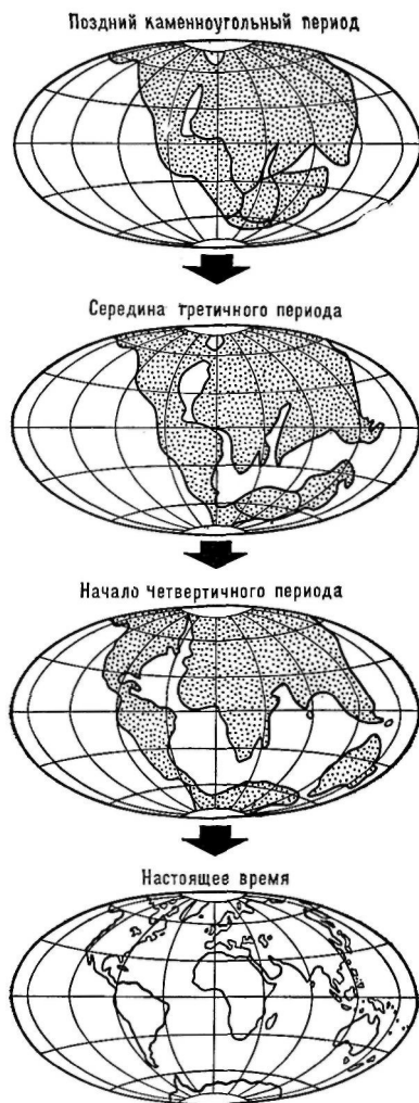
Рис. 2. Перемещение материков по Вегенеру.
