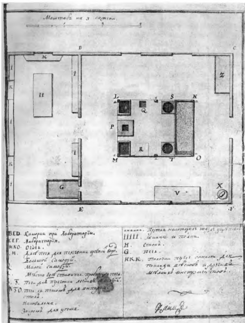
План Химической лаборатории с объяснениями, писанными рукой М. В. Ломоносова (март 1745 г.)
