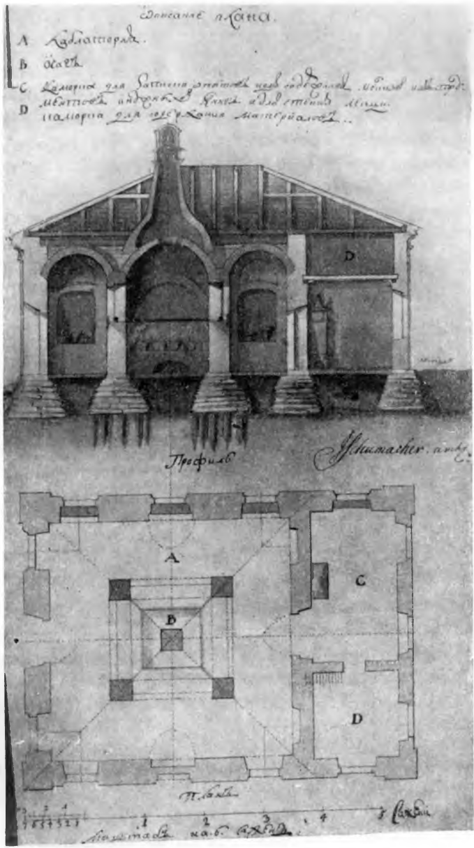
Разрез и план Химической лаборатории (1748 г.) Архив Академии Наук СССР
