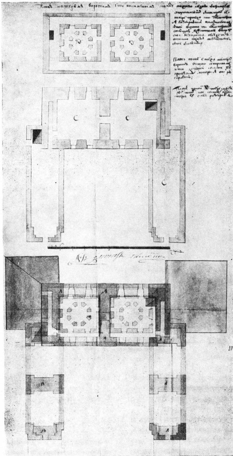
Д. Ухтомский. Обмерные чертежи шести ворот Всехсвятского моста. План
