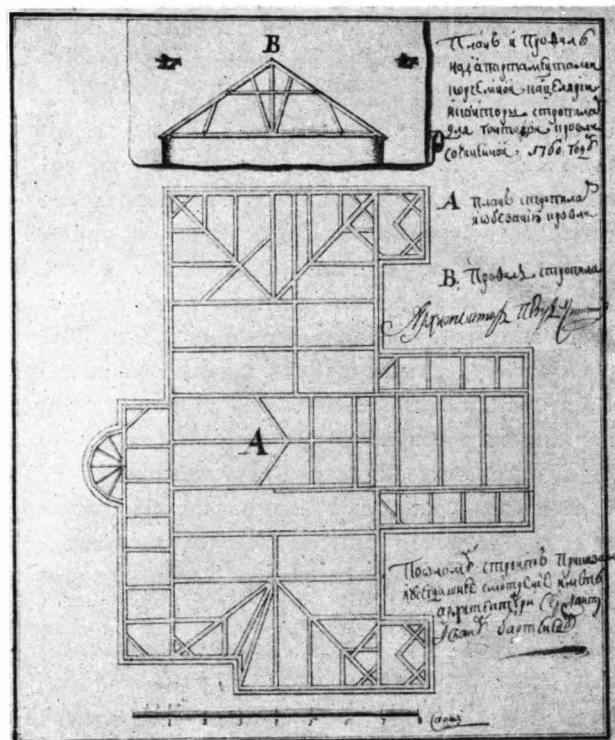
П. Никитин. Проект кровли над зданием Корчешной канцелярии
