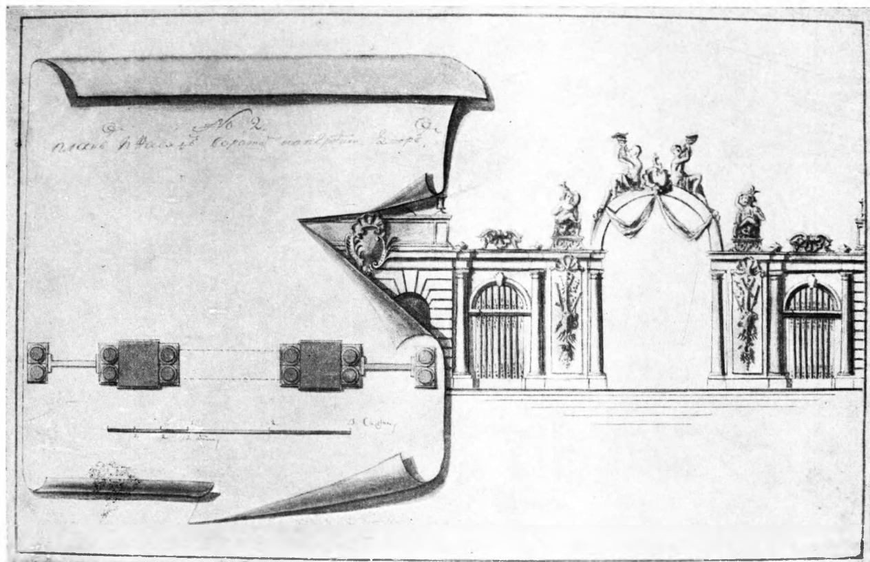
Усадьба Н. Трубецкого в Нескучном. Ворота на парадный двор
