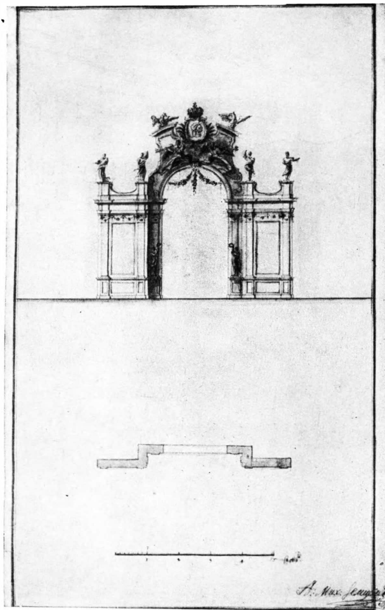
М. Земцов. Проект Яузских триумфальных ворот около Анненгофского дворца (1742)
