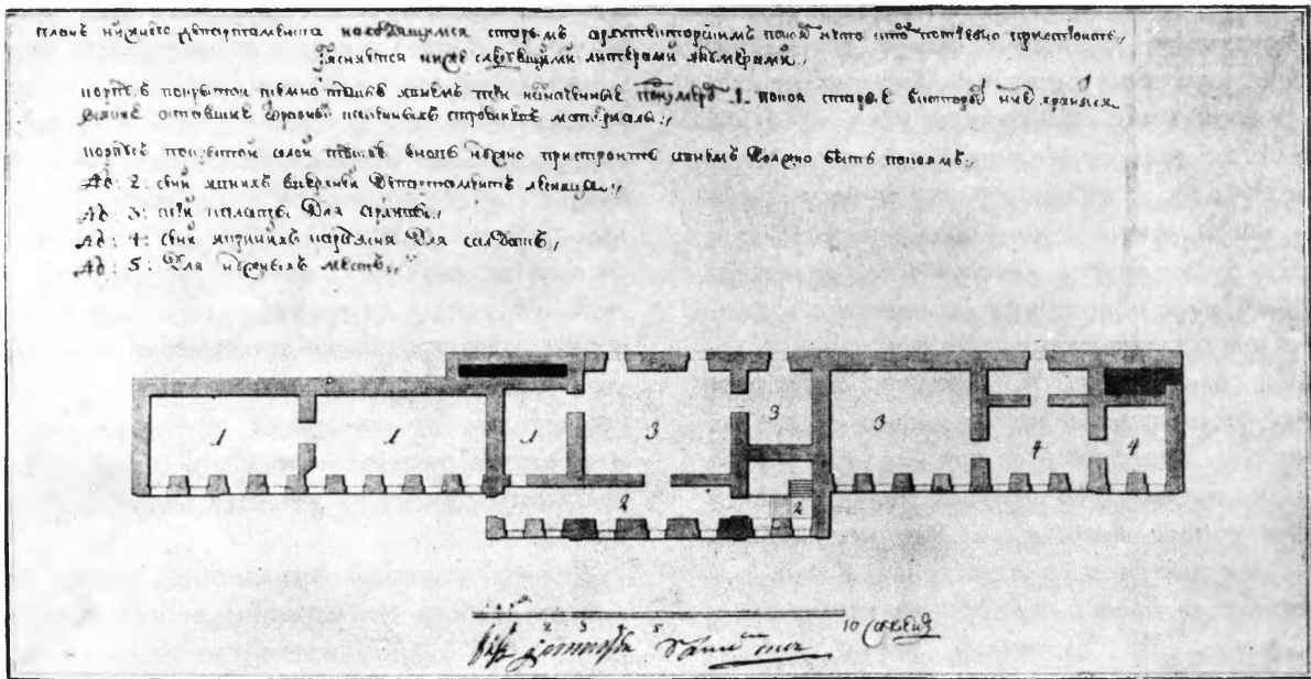
Д. Ухтомский. Проект перестройки здания архитектурной школы. План нижнего этажа
