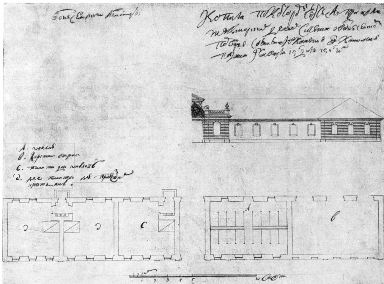
С. Яковлев. Проект конюшенного двора Вознесенского подворья
