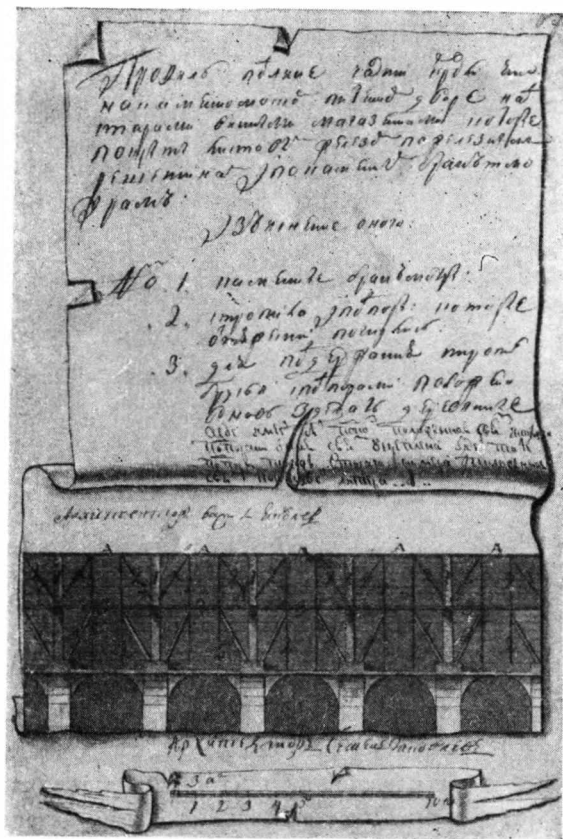
С. и В. Яковлевы. Профиль части кровли на магазинах Каменномоетского питейного двора
