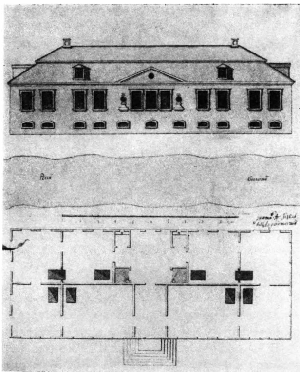
А. Расловлев. Проект Путьского дворца в Новгороде (1747), 1-й вариант
