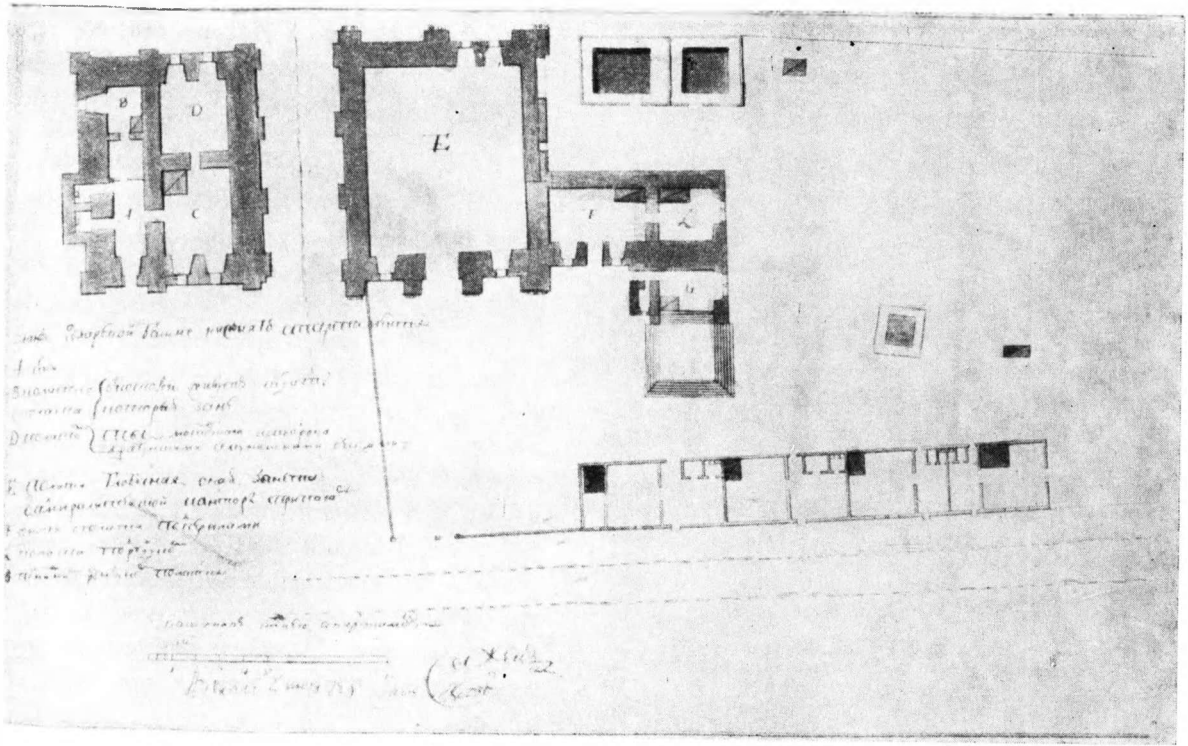
С. Яковлев. План нижнего этажа Сухаревой башни
