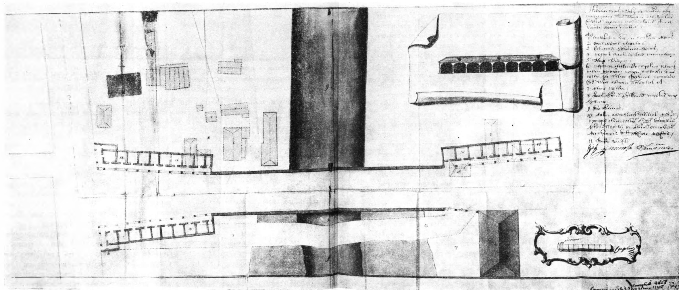
Д. Ухтомский. Проект ансамбля торговых рядов около Кузнецкого моста (1-й вариант) (1756)
