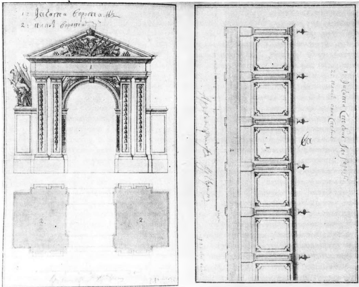
И. Мичурин. Проект здания Главного комиссариата около Красных ворот. Ограда и ворота (40-е годы XVIII вв.)
