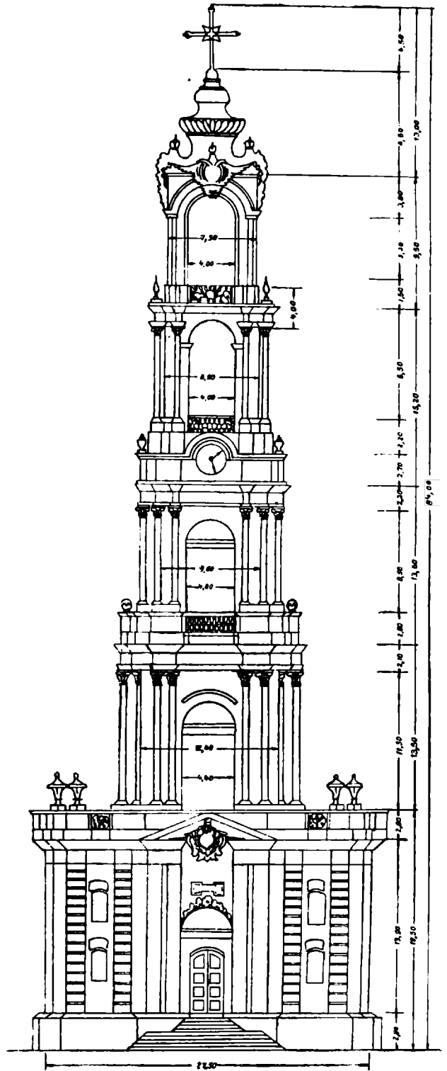
Колокольня Троице-Сергиевой лавры. Схематический чертеж фасада с указанием размеров, выполненный арх. Г. Ф. Сенатовым
