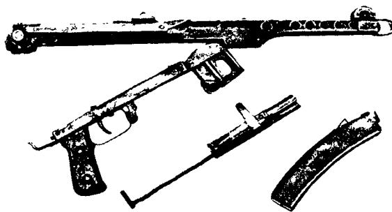
Части пистолета-пулемета.
