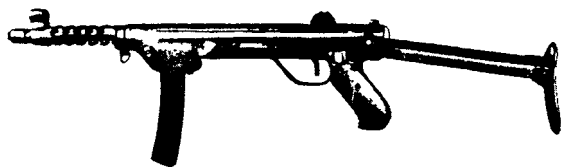
Пистолет-пулемет DUX59.
