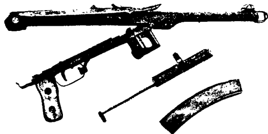
Части пистолета-пулемета.
