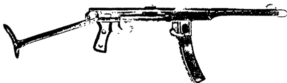
Вид справа. Приклад откинут. Проходил полигонные испытания в 1942—1943 гг.
