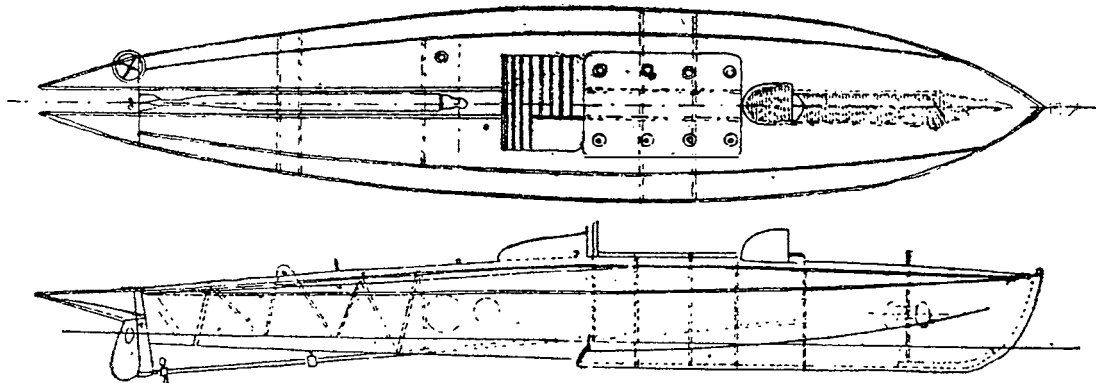
Чертеж английского быстроходного торпедного катера (С.М.В.). Вид сверху и разрез.
