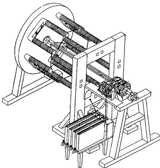
Магнитный аппарат из восьми стержней, расположенных симметрично на подвижном диске (машина Якоби).
