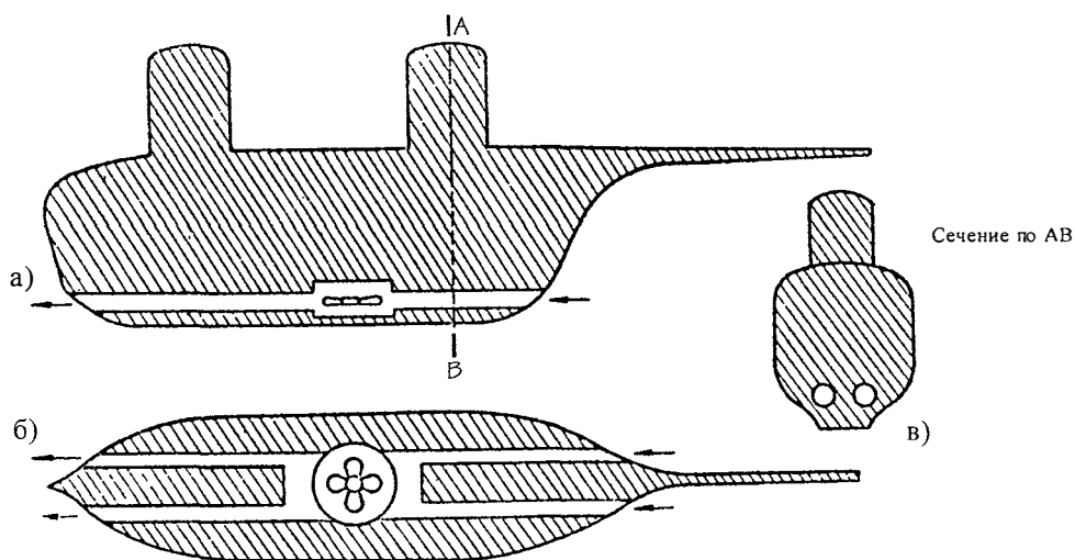
«Водогон» конструкции А. А. Саблукова: а — вид сбоку; б — вид в плане; в — поперечное сечение.
