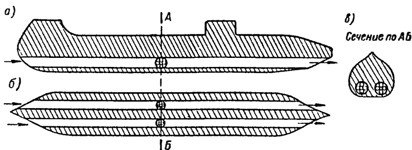
Проект подводной лодки с системой водопротоков и «внутренними» винтами: а — вид сбоку; б — вид в плане; в — поперечное сечение.
