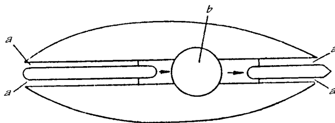
Схема гидрореактивного двигателя С. А. Бурачека.
