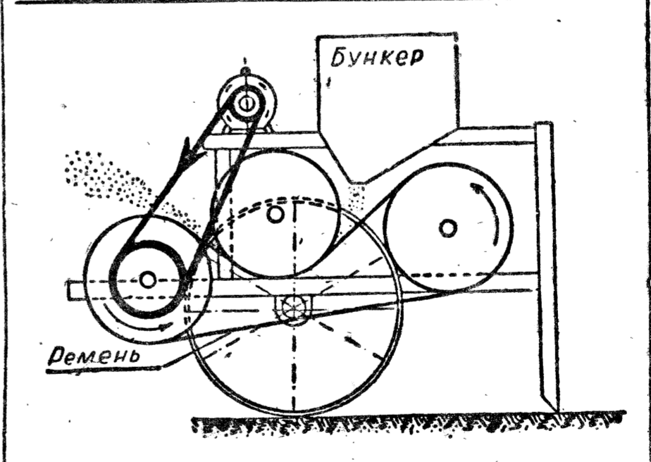
Схема устройства зернопульта. Зерно из бункера попадает на ленту, натравливаю вокруг трех шкивов. Вращением шкивов зерно бросается на определенное расстояние, очищаясь по пути от сора.
