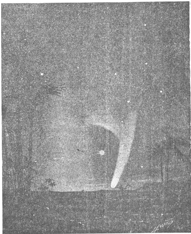
Комета 1910 года, как она была видна из Египта; рядом видна Венера и столб света, так называемый зодиакальный свет.
