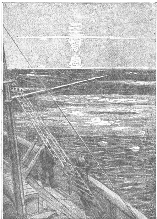
Видение, или мираж, на море. Корабль отражается в небе, словно в зеркале.
