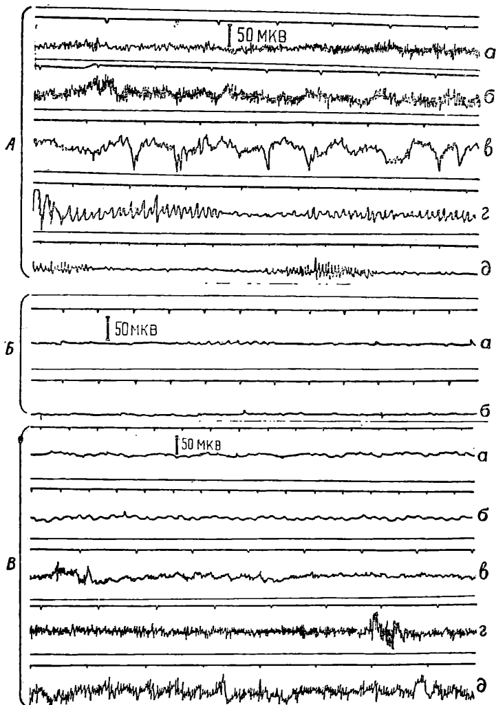
Электрэнцефалограмма кошки в период умирания от потери крови (А), во время клинической смерти (Б) и в ходе восстановления деятельности коры больших полушарий в период оживания (В). Время отмечается в секундах. 50 мкв (микровольт) — масштаб колебаний биопотенциала. Пояснение в тексте.
