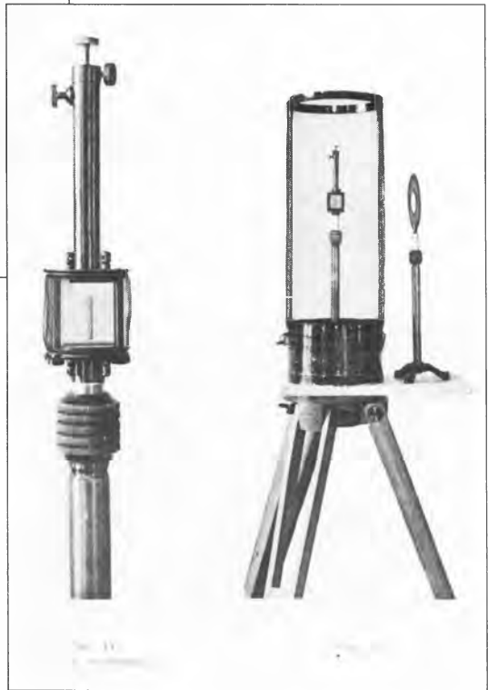
Портативный фонометр Лебедева—Зёрнова (общий вид).
